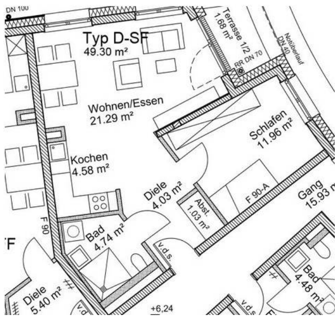
Grundriss
